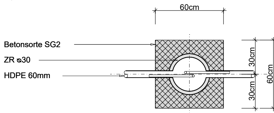
Querschnitt A-A
